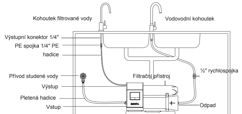
Obr.5 Instalační schéma
