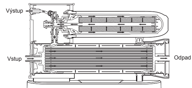
Obr.2 Princip výroby vody
